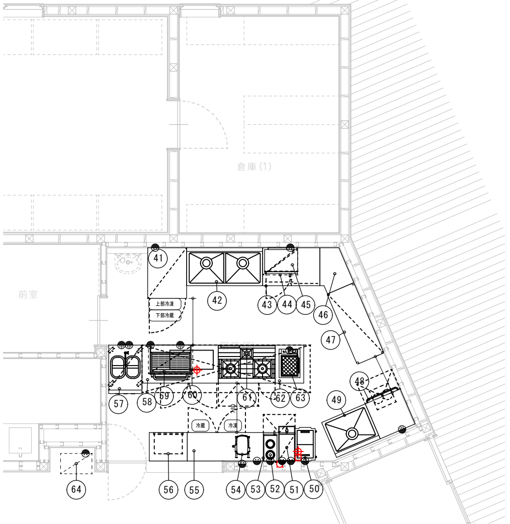
テイクアウトテナント厨房機器配置図 1/30
