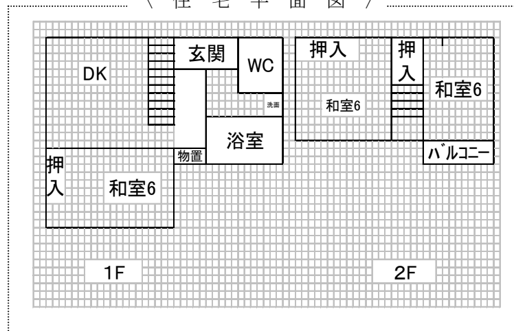
〈 住 宅 平 面 図 〉
