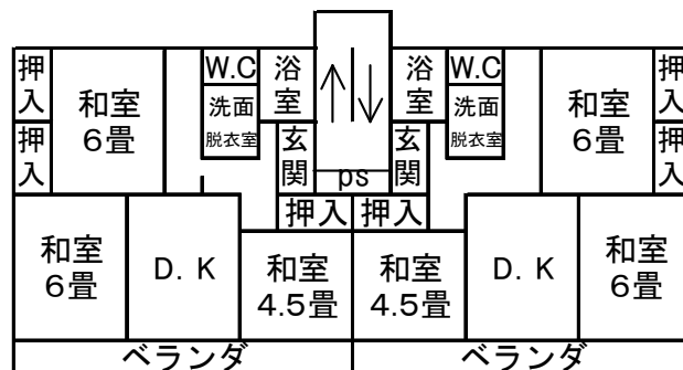
<住宅平面図>
