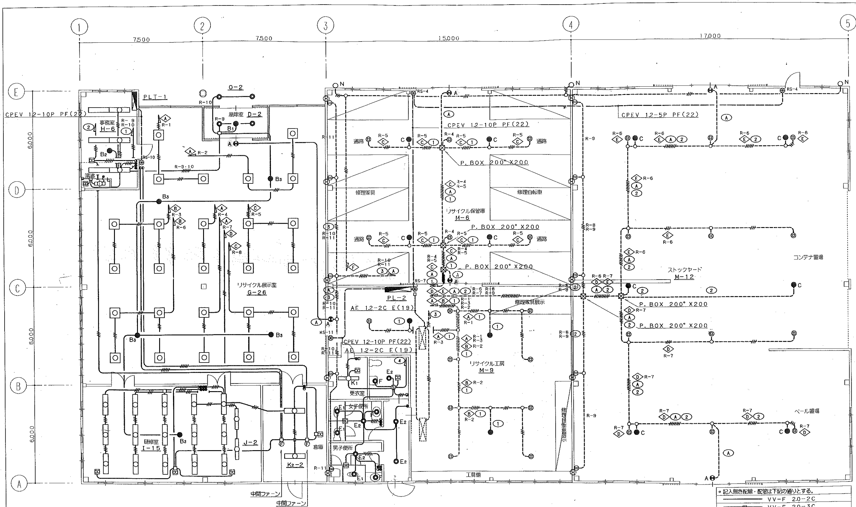
平面図 S=1/100
