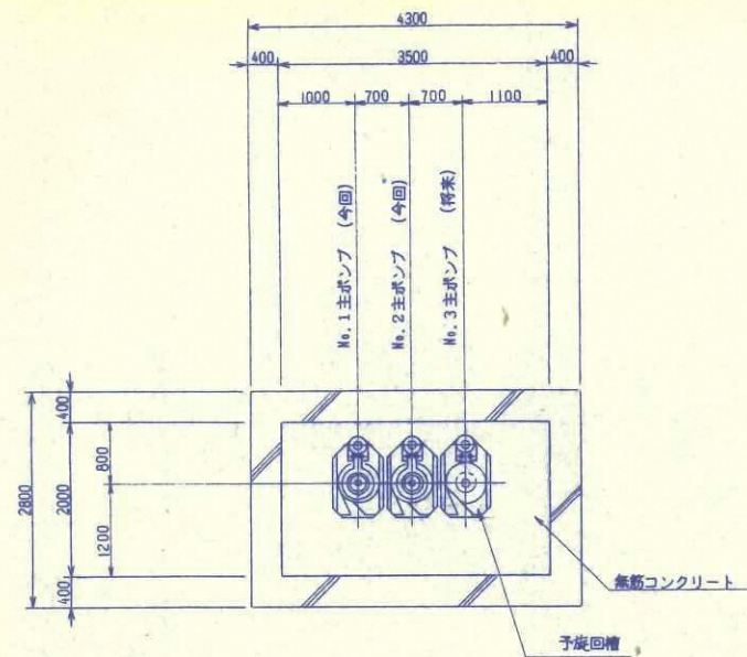
ポンプ井平面図 (S=1/50)
