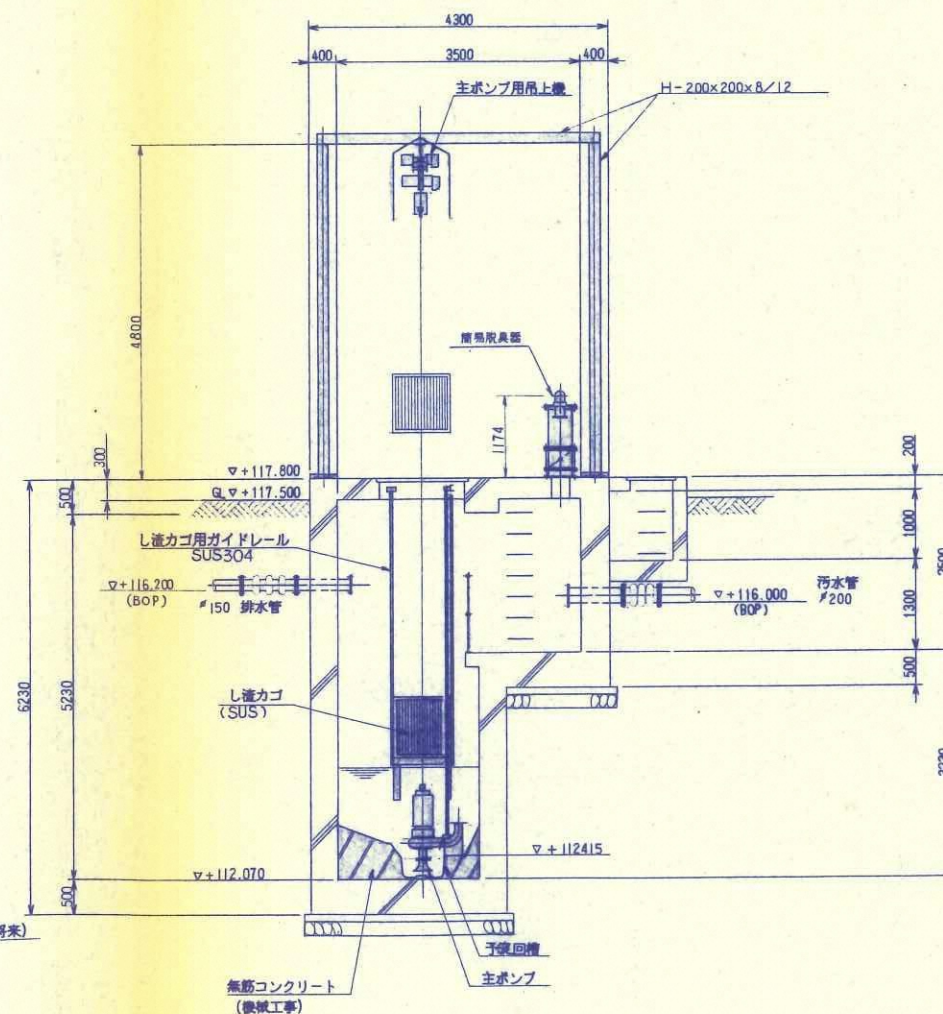
B-B断面図 (S=1/50)
