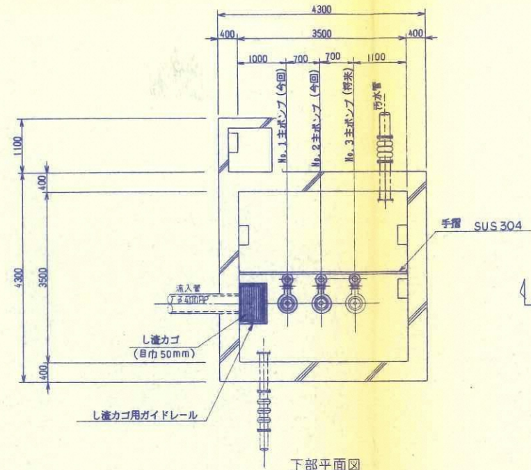
下部平面図 (S=1/50)
